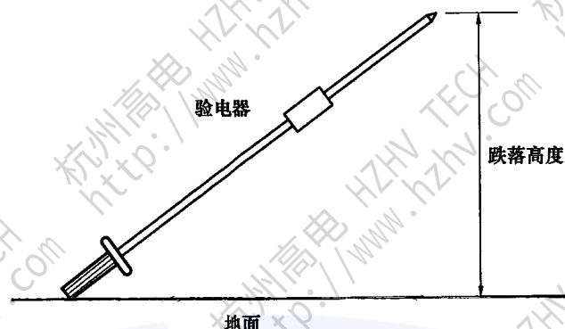
图 27 抗跌落试验——对角线位置
