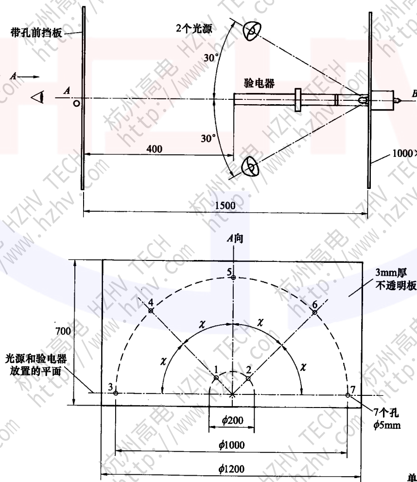
图 15 光指示信号的清晰可辨性试验布置
