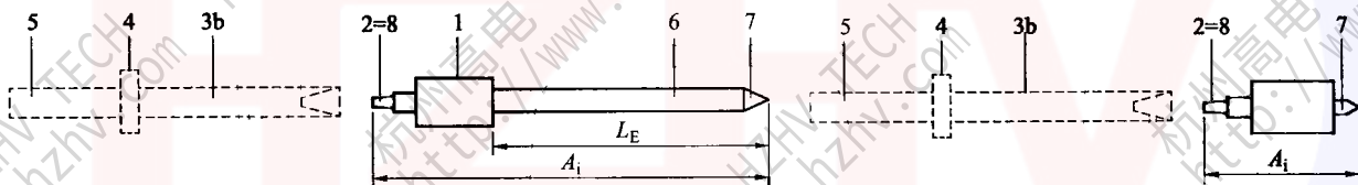
a) 有接触电极延长段的分体式验电器
