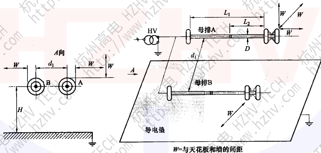
图 5 试验布置图
