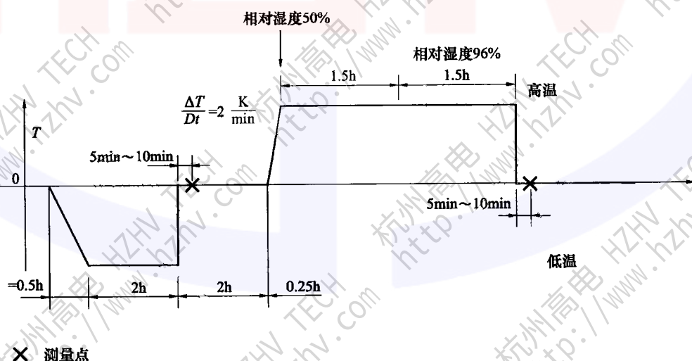
图 28 试验周期与气候的关系曲线
