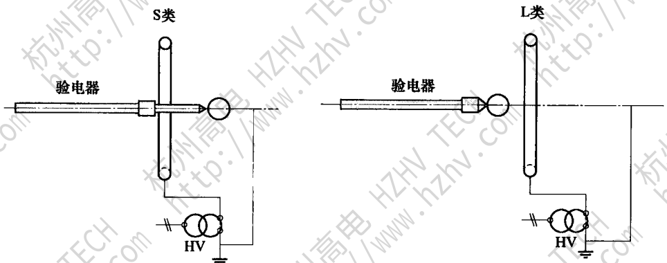
图 12 采用球和环电极的反相干扰电场影响的测试布置
