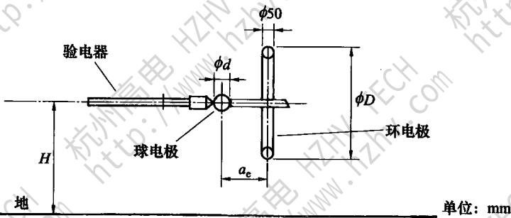
图 4 球电极在环电极之前的试验布置
