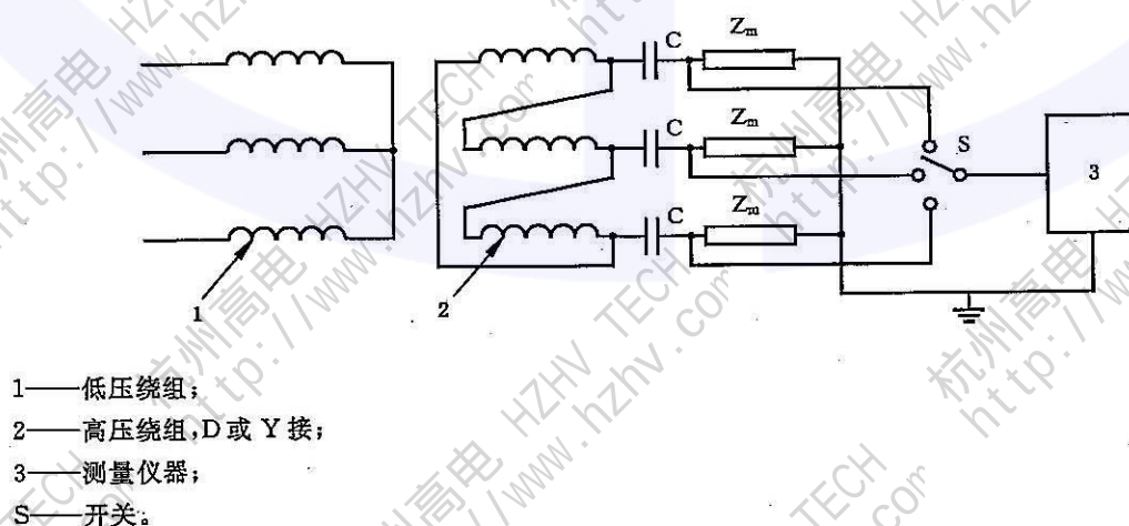
图 2 三相变压器局部放电试验的基本测量线路
