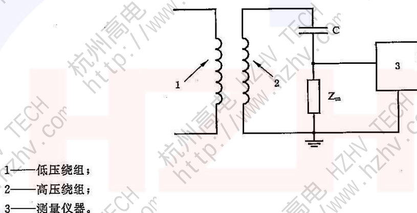
图 1 单相变压器局部放电试验的基本测量线路
