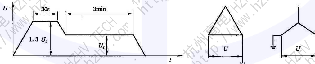
图 4 局部放电特殊试验的施加电压方式
