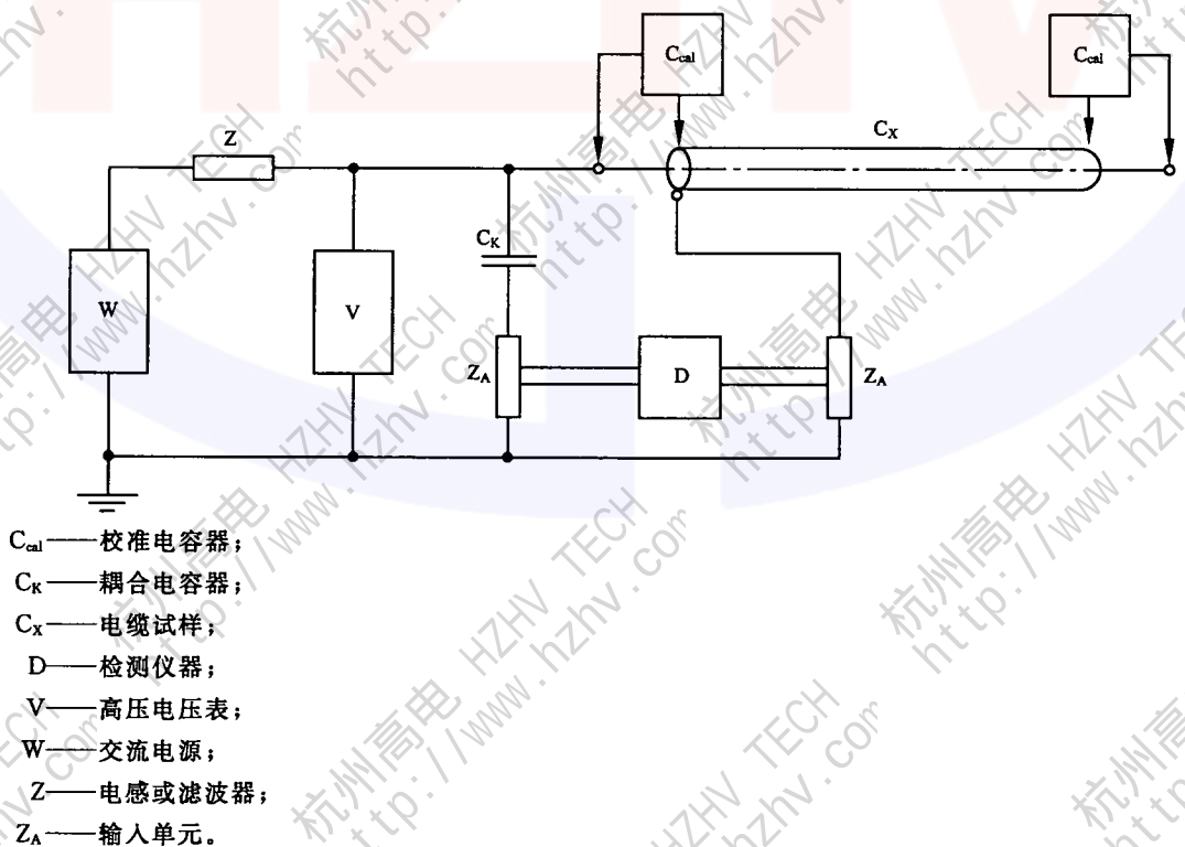
图3 电桥线路
