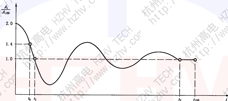
图 B.3 t_1 与 t_2 间有负的和正的叠加的双脉冲曲线(3型)
