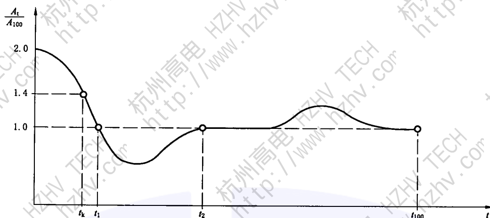
图 B.2 t_1 与 t_2 间有负叠加的双脉冲曲线图(2型)
