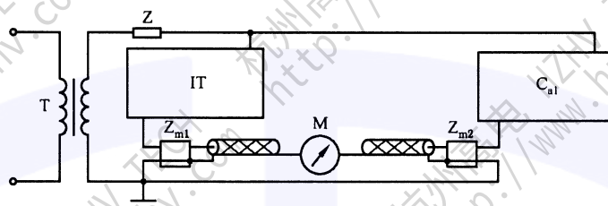
c) 平衡法回路
