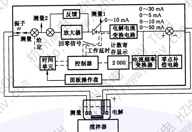
图 21 YS-2 型微库仑仪分析系统原理框图
