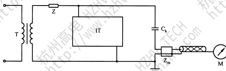
b) 并联回路
