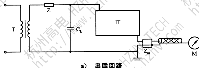
图 12 局部放电测量的试验电路示例
