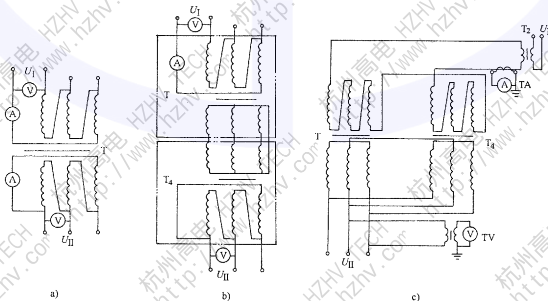
T——试品； T_4 ——辅助变压器； T_2 ——中间变压器；A——电流表；V——电压表；TA——电流互感器；TV——电压互感器； U_1 ——供试验用的单相交流电源； U_{II} ——供试验用的三相交流电源。
