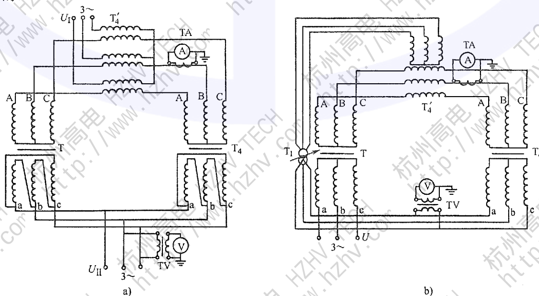
图 14 相互负载法原理接线图
