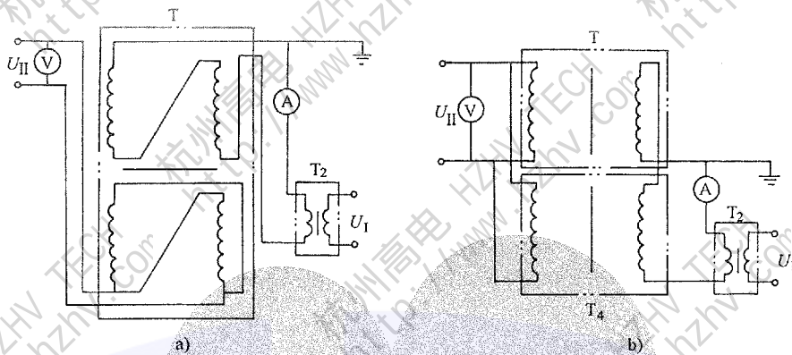
T——试品；T 2 ——中间变压器；T 4 ——辅助变压器；A——电流表； V——电压表；U I 、U II ——供试验用的单相交流电源。
