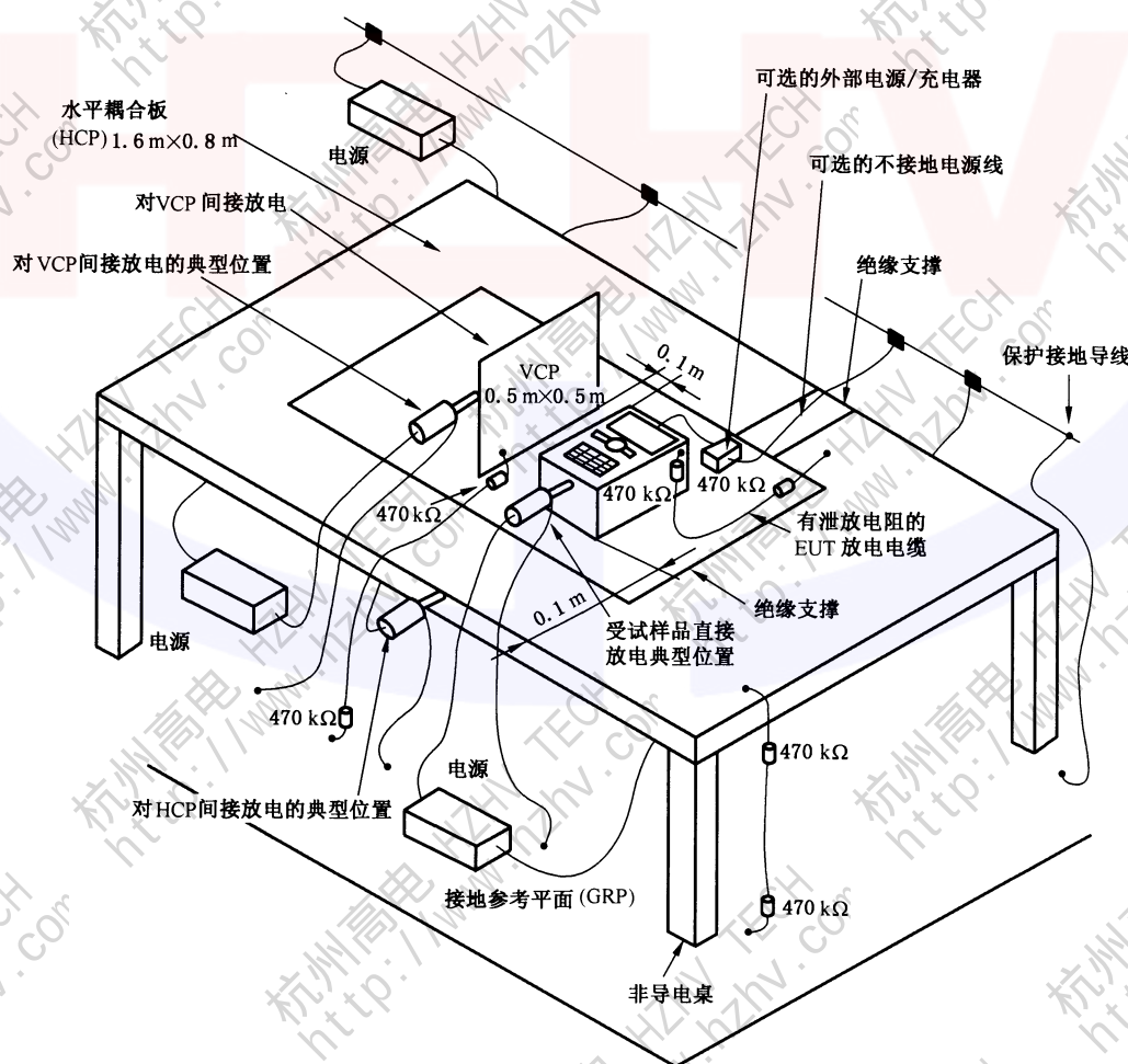
图 6 不接地台式设备试验布置实例
