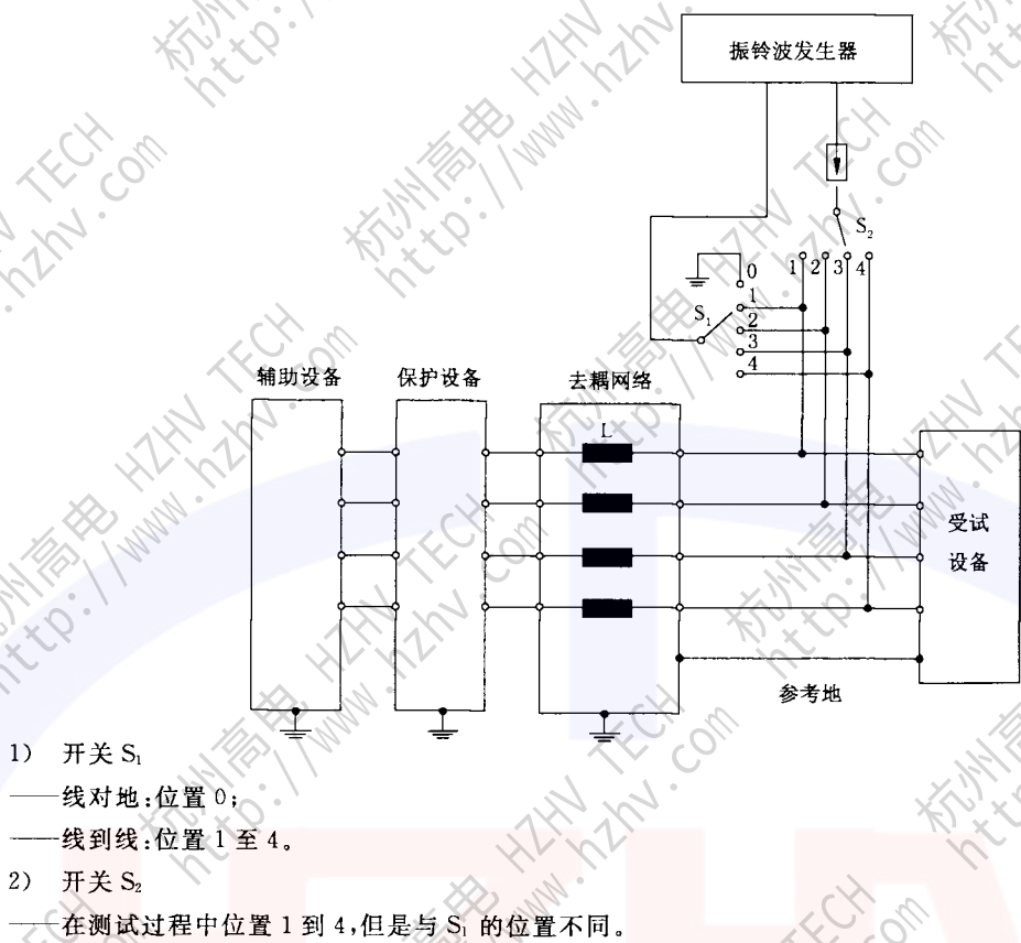
图 10 非屏蔽不对称互连线避雷器耦合试验布置示例(线对线和线对地)
