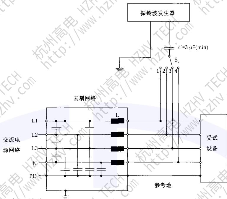
图 8 交流电源线(三相)电容耦合试验布置示例(L3 线对地)
