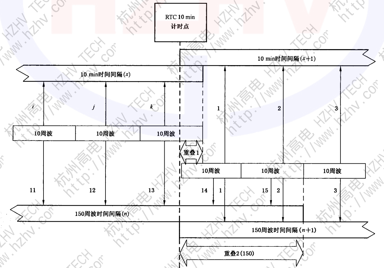
图 2 A 类累积时间间隔的同步
