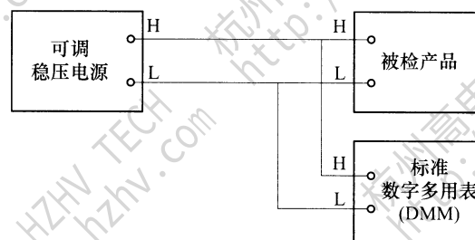
图2 直接比较法接线
